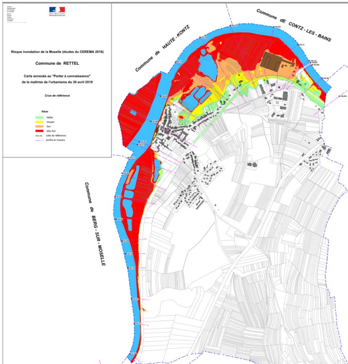
Cartographie de l'aléa inondation (crue de référence) de la Moselle, CEREMA – 2018
